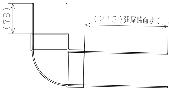
S字トラップ接続配管図 (VU75) ※本部品は付属してありません
